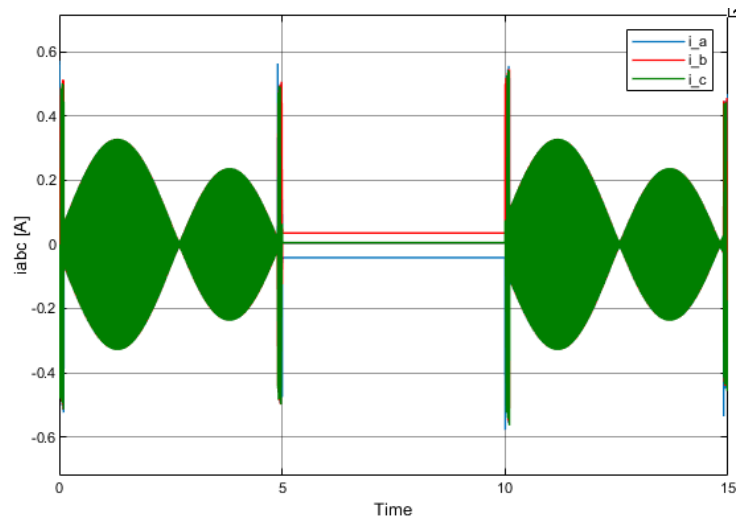
Figura 87: Curvas de i_{abc} con \omega_{n\_modulador} = 18000 \text{ rad/s}
