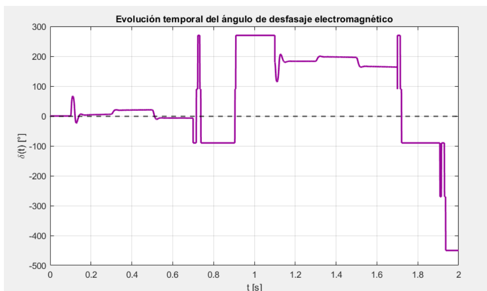
Figura 26 Evolución temporal del ángulo \delta(t)
