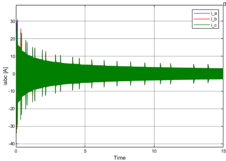
Figura 86: Curvas de i_{abc} con \omega_{n\_modulador} = 6000 \text{ rad/s}
